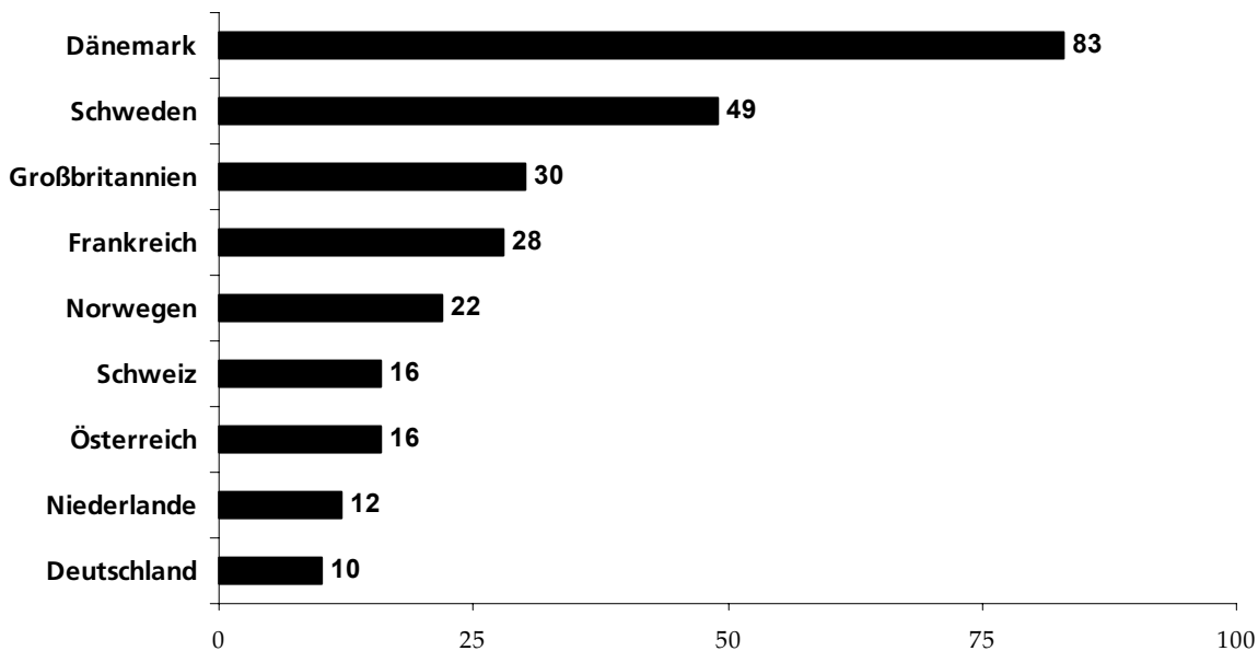
Morphinverbrauch in Kilogramm pro 1 Million Einwohner (1995,WHO)
